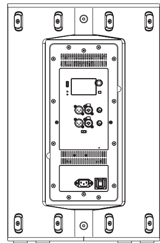
背面図
