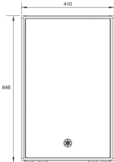
正面図
