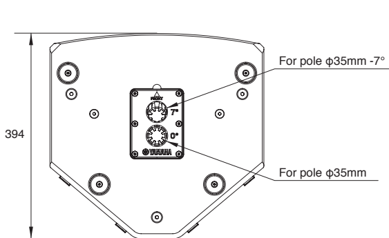
底面図
