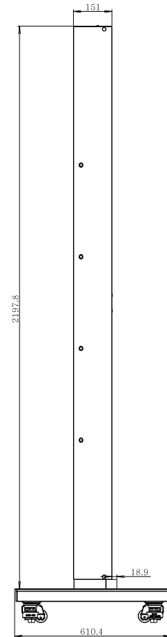
[ SIDE ]
